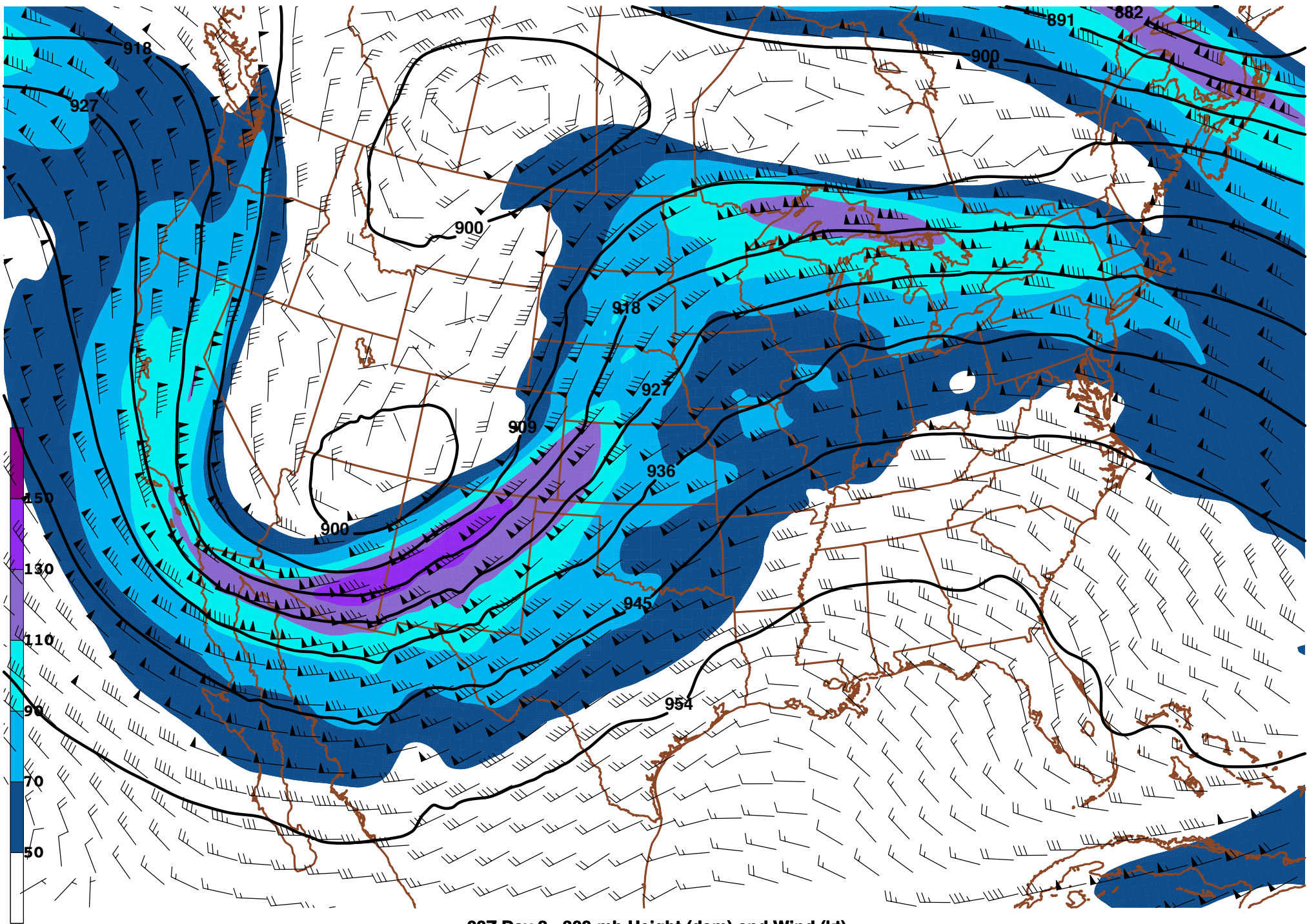
00Z Day 2 - 300-mb Height (dam) and Wind (kt)
