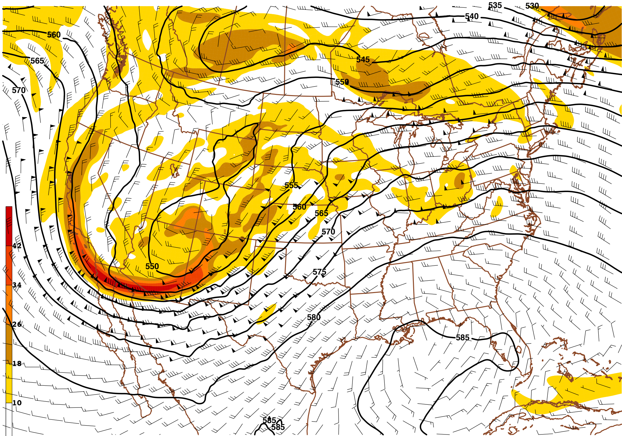
00Z Day 2 - 500-mb Abs. Vort. ( s \cdot 10^{-5} ), Height (dam), and Wind (kt.)
