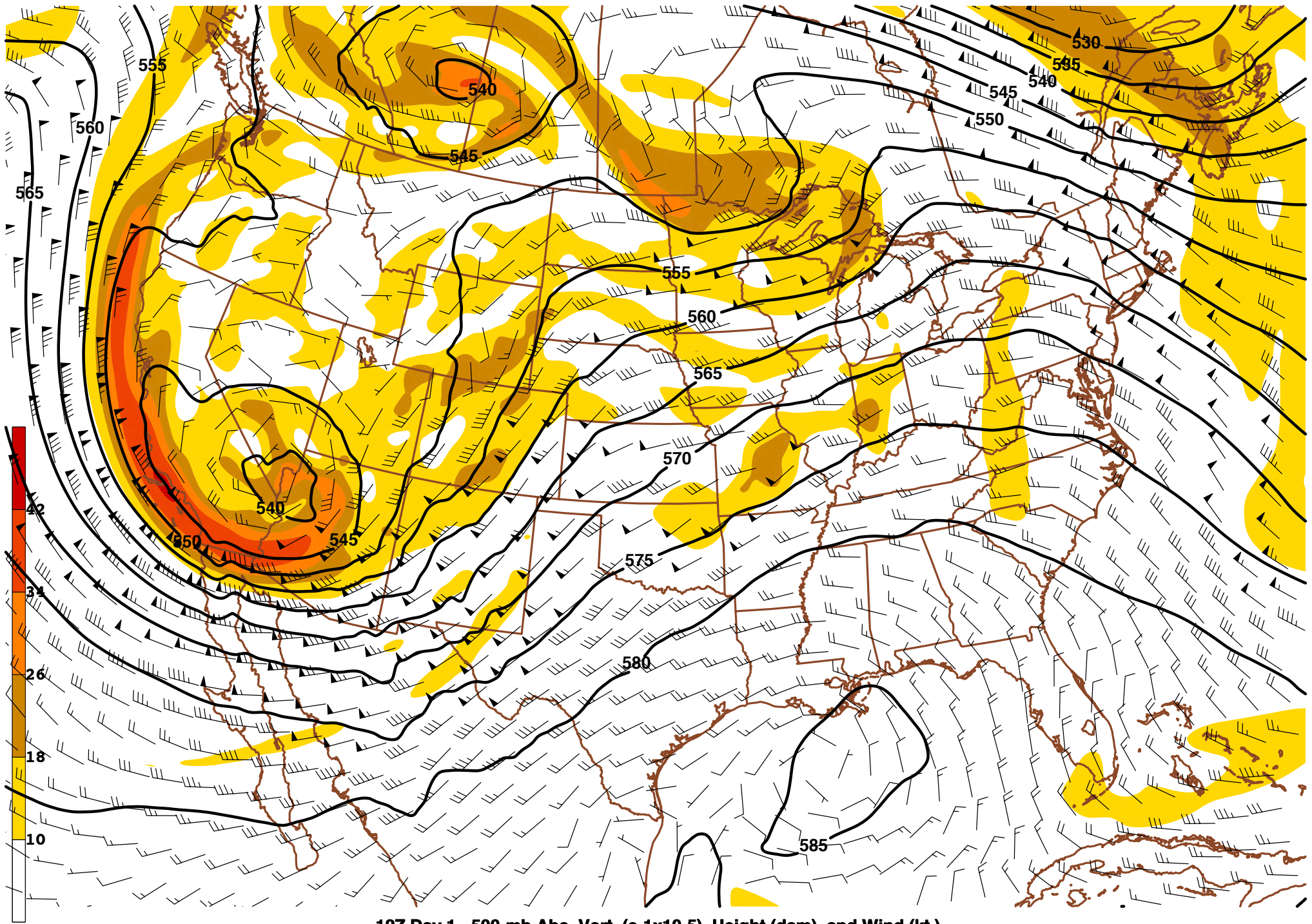
12Z Day 1 - 500-mb Abs. Vort. ( s \cdot 10^{-5} ), Height (dam), and Wind (kt.)
