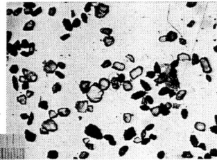
05-11b, U35Z-58 Grain 67
