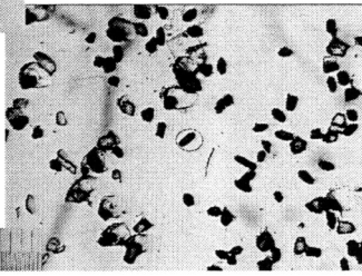
05-13b, U35Z-62 Grain 32
