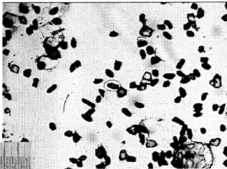
05-13b, U35Z-62 Grain 37
