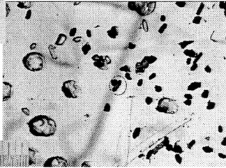
05-13b, U35Z-62 Grain 43
