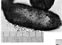
05-13b, U35Z-62 Grain 87
