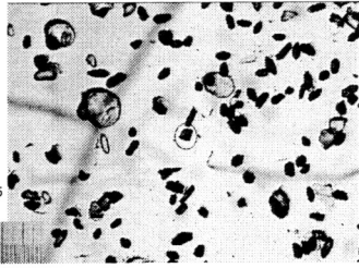
05-13b, U35Z-62 Grain 105
