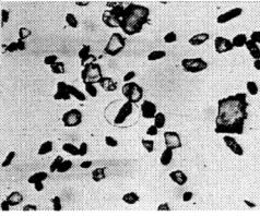
05-11b, U35Z-58 Grain 59
