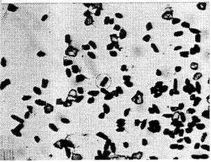
05-13b, U35Z-62 Grain 117
