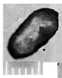
05-04a, U35Z-49 Grain 79
