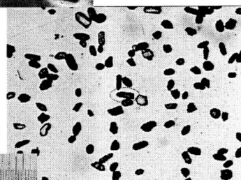
05-04a, U35Z-49 Grain 64
