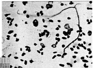
05-13b, U35Z-62 Grain 111
