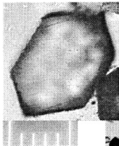
05-10a, U35Z-55 Grain 39
