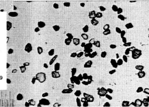
05-11b, U35Z-58 Grain 69
