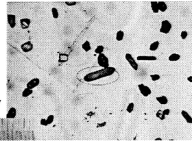
05-07a, U35Z-52 Grain 57
