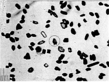
05-04a, U35Z-49 Grain 87
