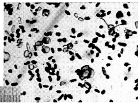
05-13b, U35Z-62 Grain 87
