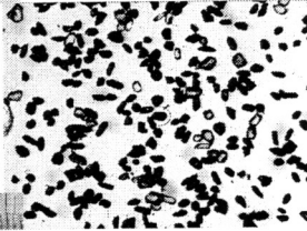
05-13b, U35Z-62 Grain 158
