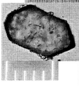
05-11b, U35Z-58 Grain 2
