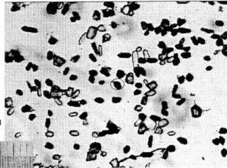
05-13b, U35Z-62 Grain 133
