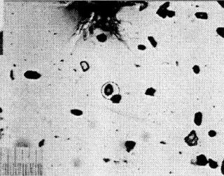
05-04b, U35Z-50 Grain 1
