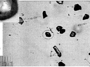
05-10a, U35Z-55 Grain 36
