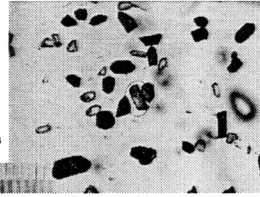
05-10a, U35Z-55 Grain 24
