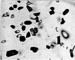
05-10a, U35Z-55 Grain 34
