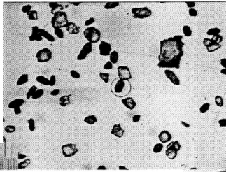
05-11b, U35Z-58 Grain 58
