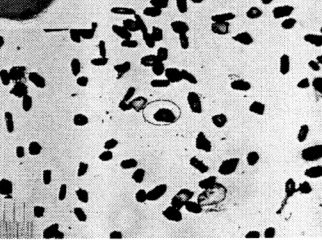
05-04a, U35Z-49 Grain 62
