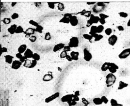
05-10a, U35Z-55 Grain 41
