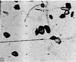
05-10a, U35Z-55 Grain 36
