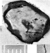
05-10a, U35Z-55 Grain 34
