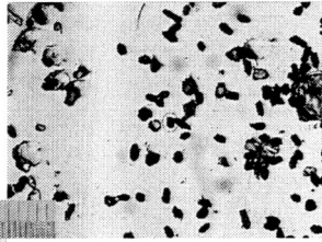
05-13b, U35Z-62 Grain 30
