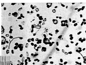
05-13b, U35Z-62 Grain 76
