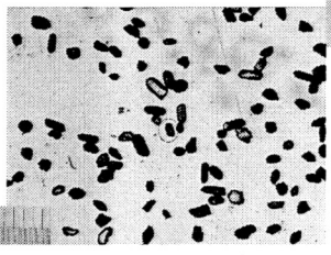
05-04a, U35Z-49 Grain 68
