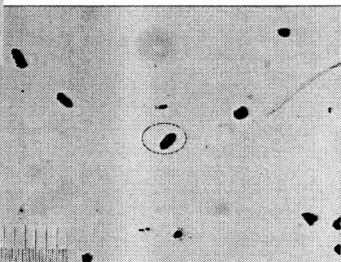
05-04a, U35Z-49 Grain 85
