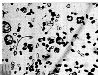
05-13b, U35Z-62 Grain 77
