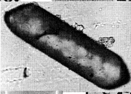
05-11b, U35Z-58 Grain 70
