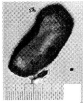
05-13b, U35Z-62 Grain 116
