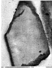
05-10a, U35Z-55 Grain 35
