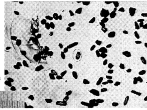
05-04a, U35Z-49 Grain 93
