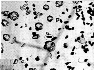
05-13b, U35Z-62 Grain 54
