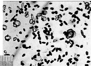
05-13b, U35Z-62 Grain 89
