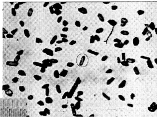
05-04a, U35Z-49 Grain 95
