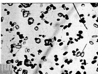
05-13b, U35Z-62 Grain 75
