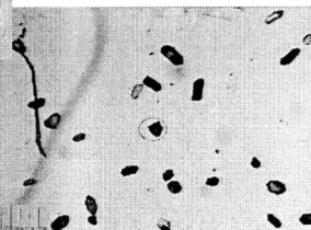
05-11b, U35Z-58 Grain 4
