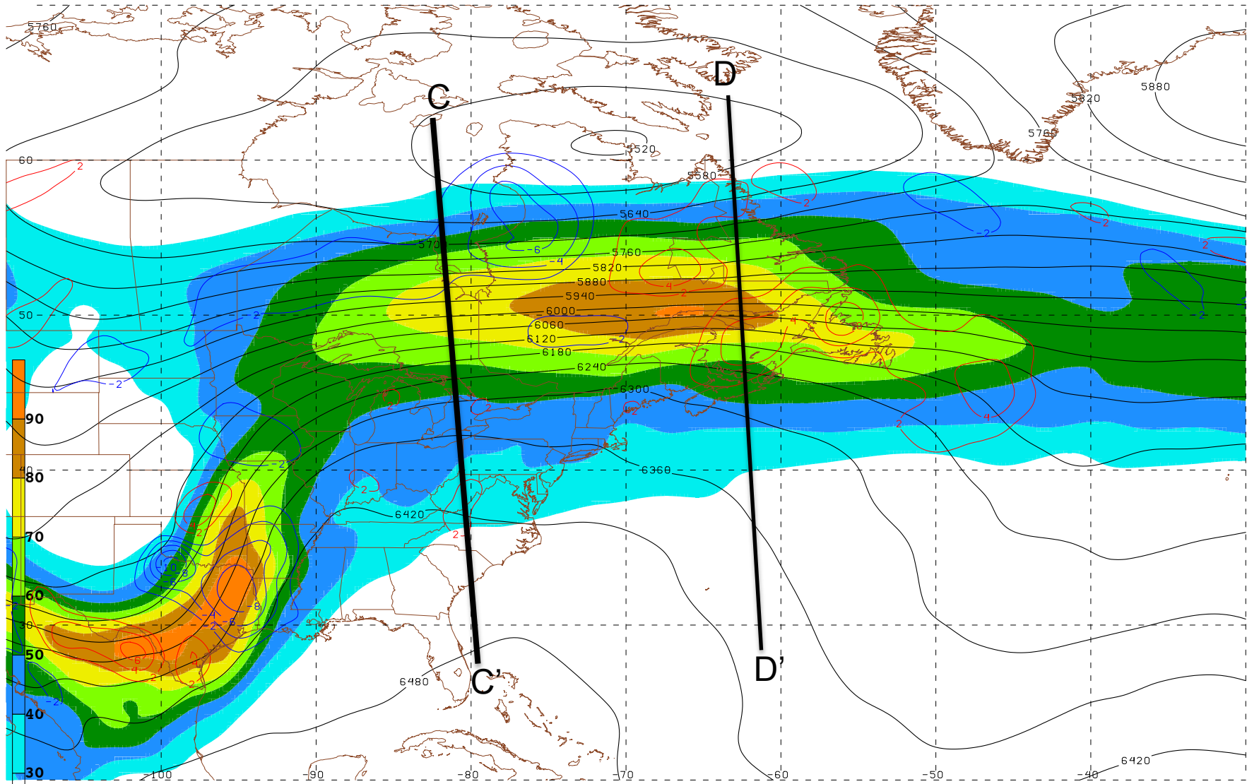
250mb geo. jet, 300-700mb thck, 400mb geo. temp. adv. 131222/0000V000
