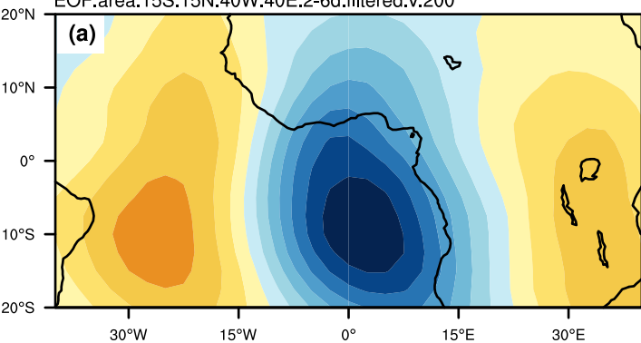
EOF.area.15S.15N.40W.40E.2-6d.filtered.v.200
