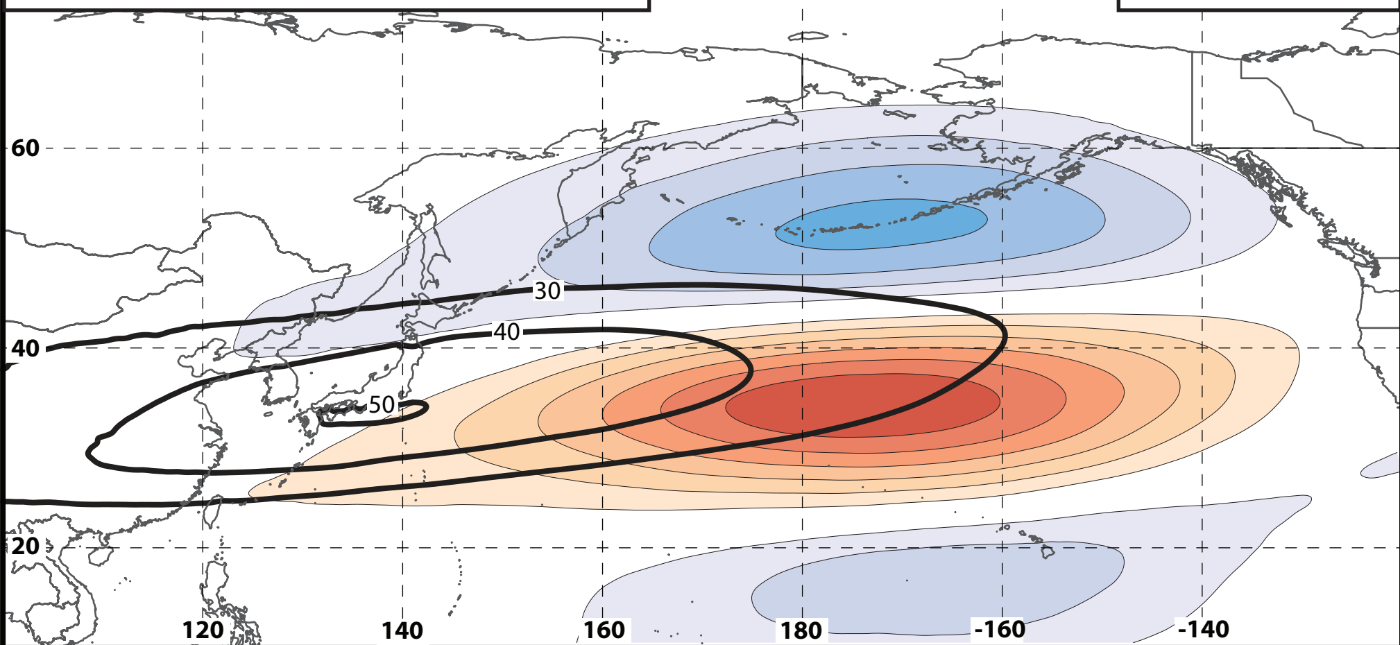
(b) EOF 2: Poleward/Equatorward Shift
