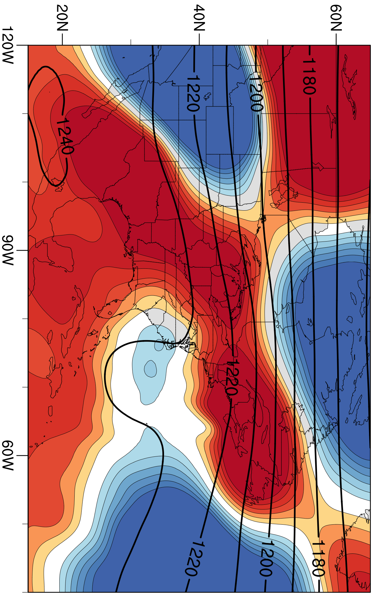
(h) EOF 8: 1%
