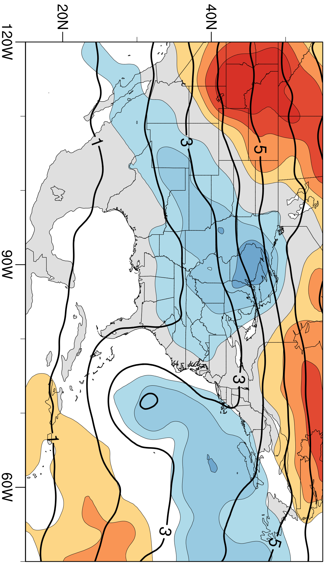
(d) EOF 4: 6.1%
